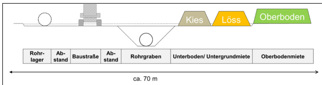
Abb. 7-1: Skizze des schematischen Regelarbeitsstreifens (RWE Power AG, verändert)
